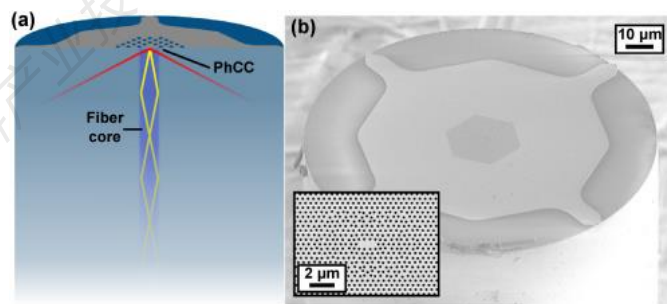
超灵敏纤维尖端传感器示意图
